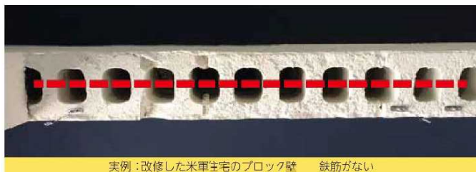
実例：改修した米軍主宅のブロック壁 鉄筋がない
