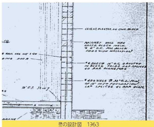
壁の設計図 1363
